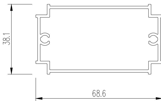
Геометрические характеристики сечения.
